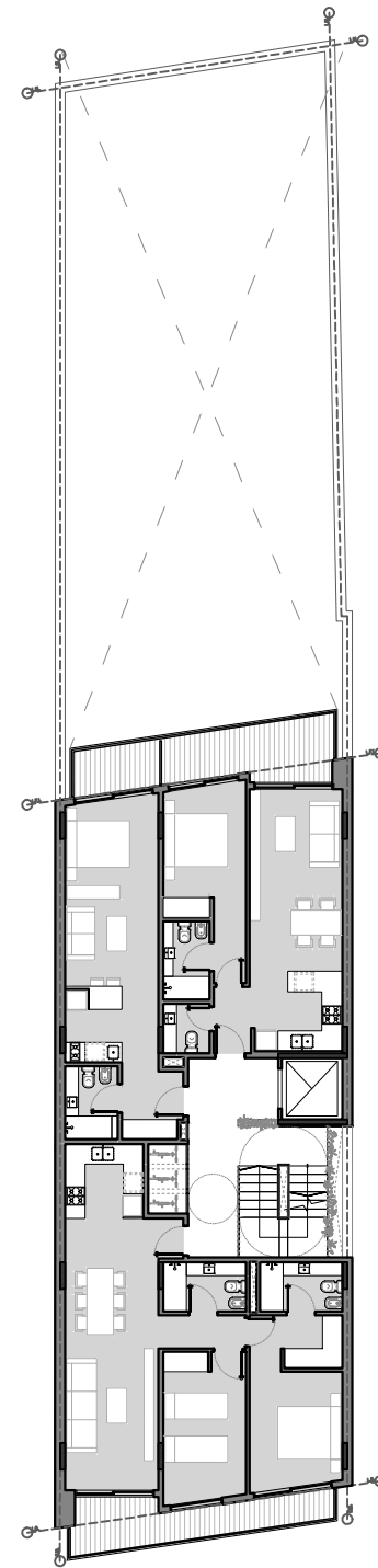
PLANTA TIPO
